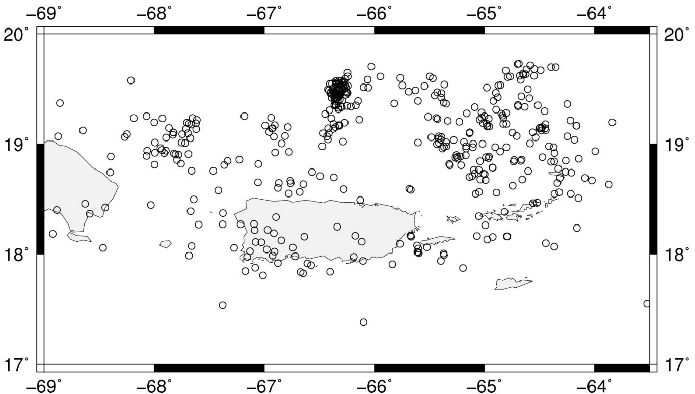
Figura 1. Mapa epicentral de los sismos localizados por la RSPR para el mes de agosto de 2015 (RSPR-UPRM).
